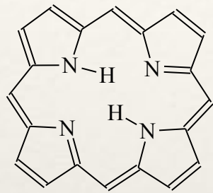
porphyrin
