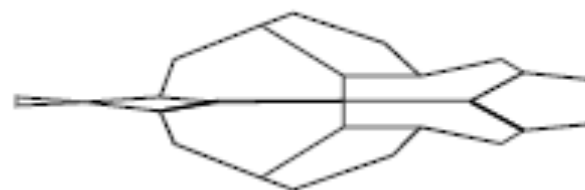
pro ( A_{1u} ), 335\text{ cm}^{-1}
