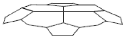
dom ( A_{2u} ), 135\text{ cm}^{-1}
