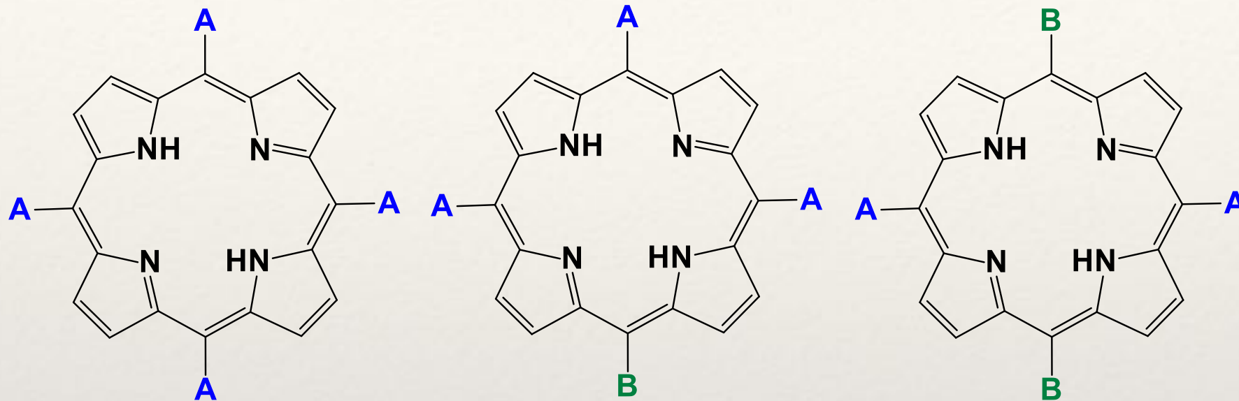
A 2 B 2 -Porphyrin
